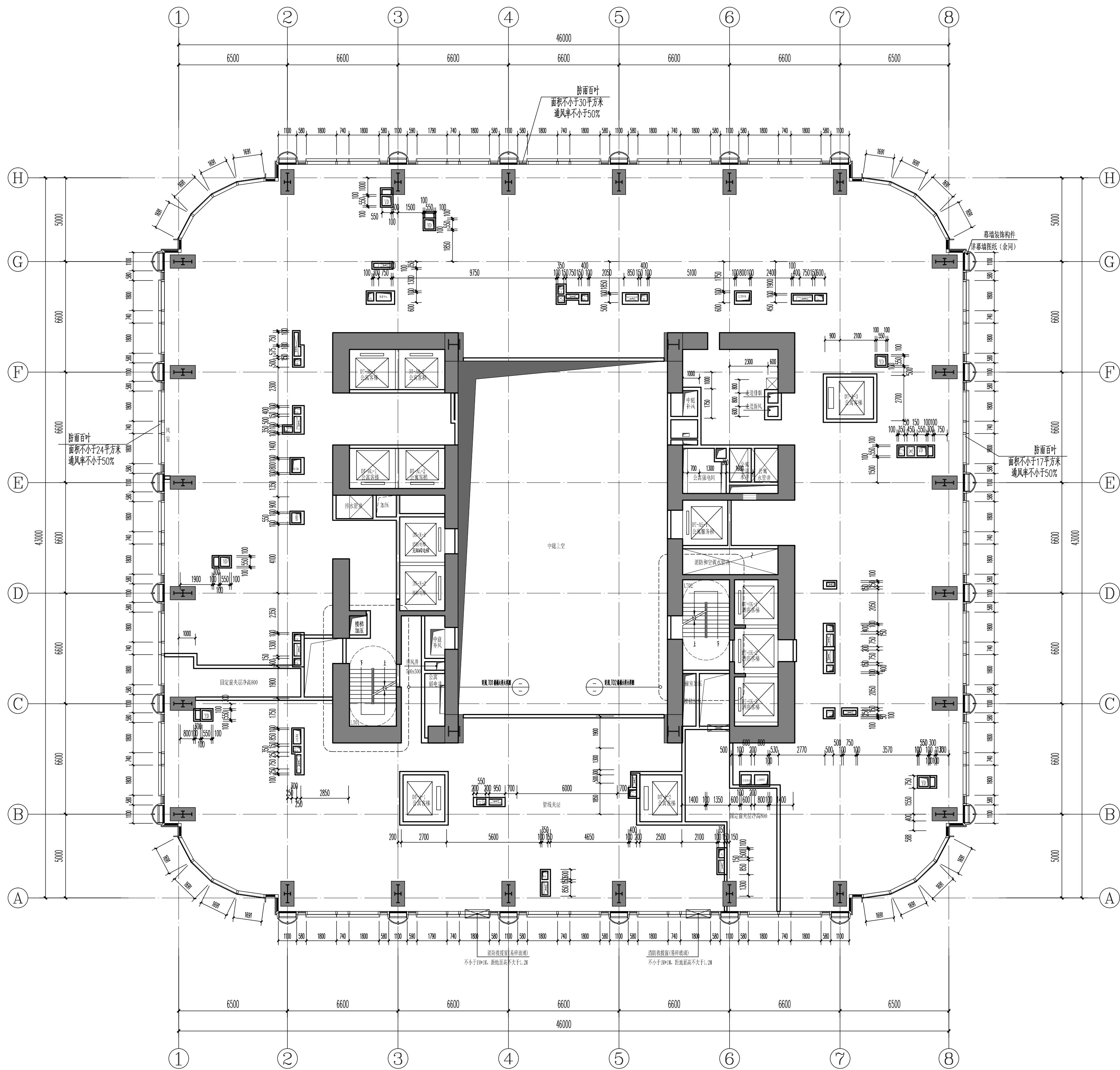
十四夹层平面图 1:150
